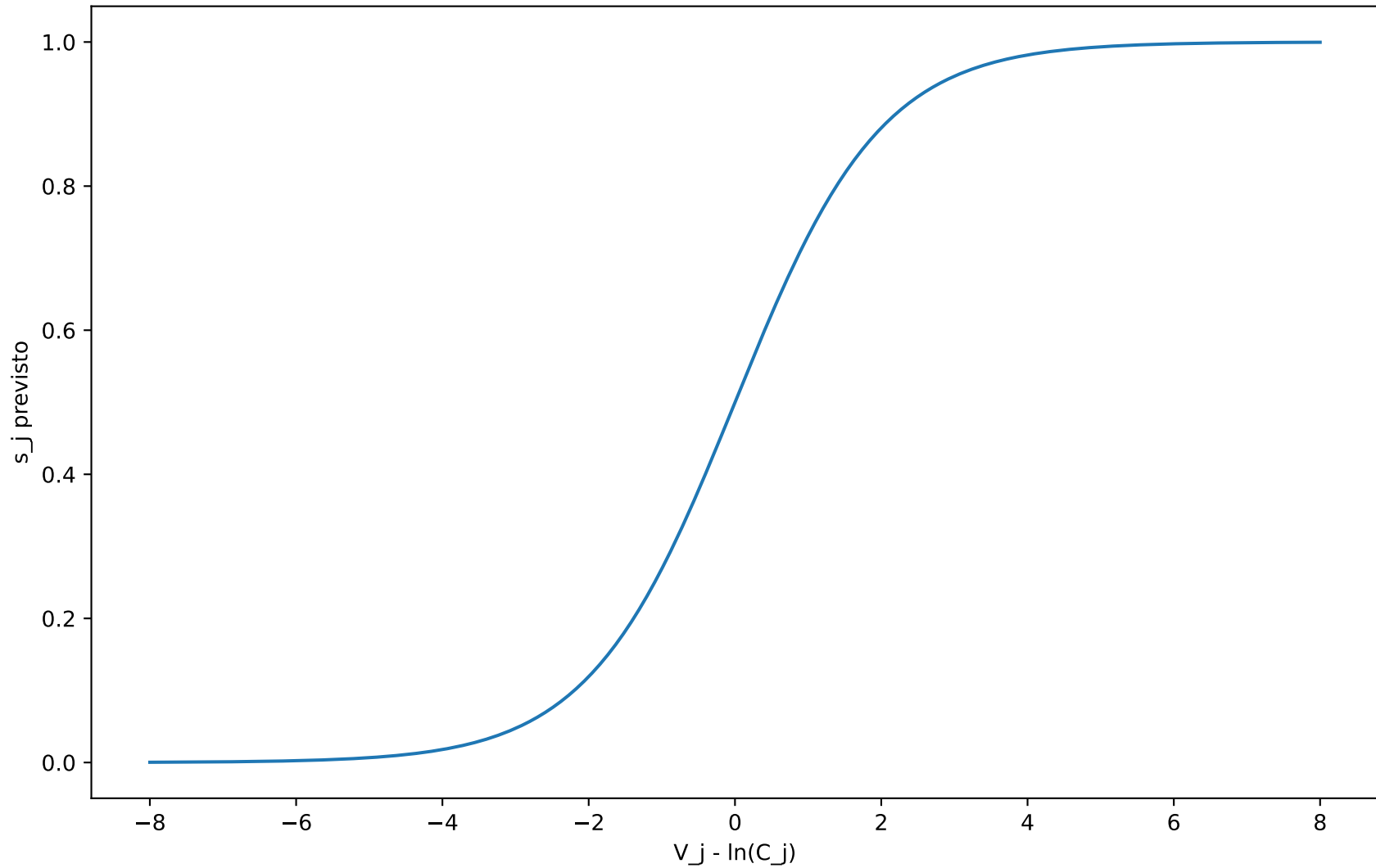
Curva clássica do logit
